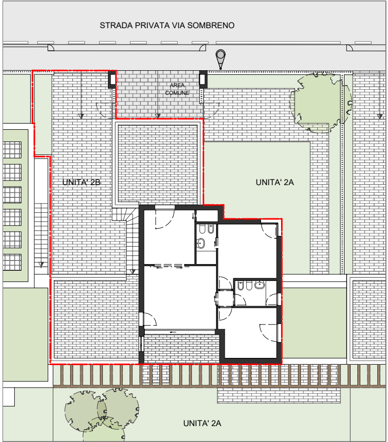
PLANIMETRIA _scala 1:250
