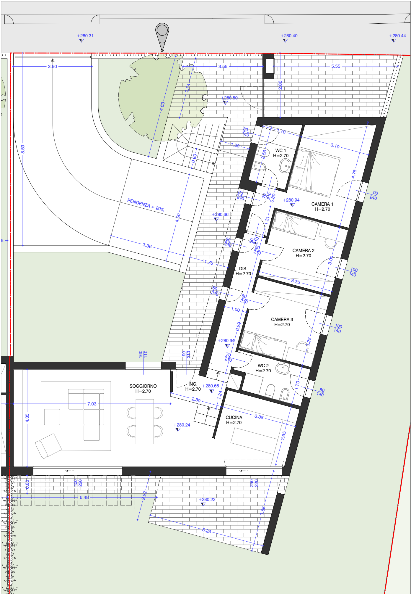
PIANO TERRA_scala 1:100
