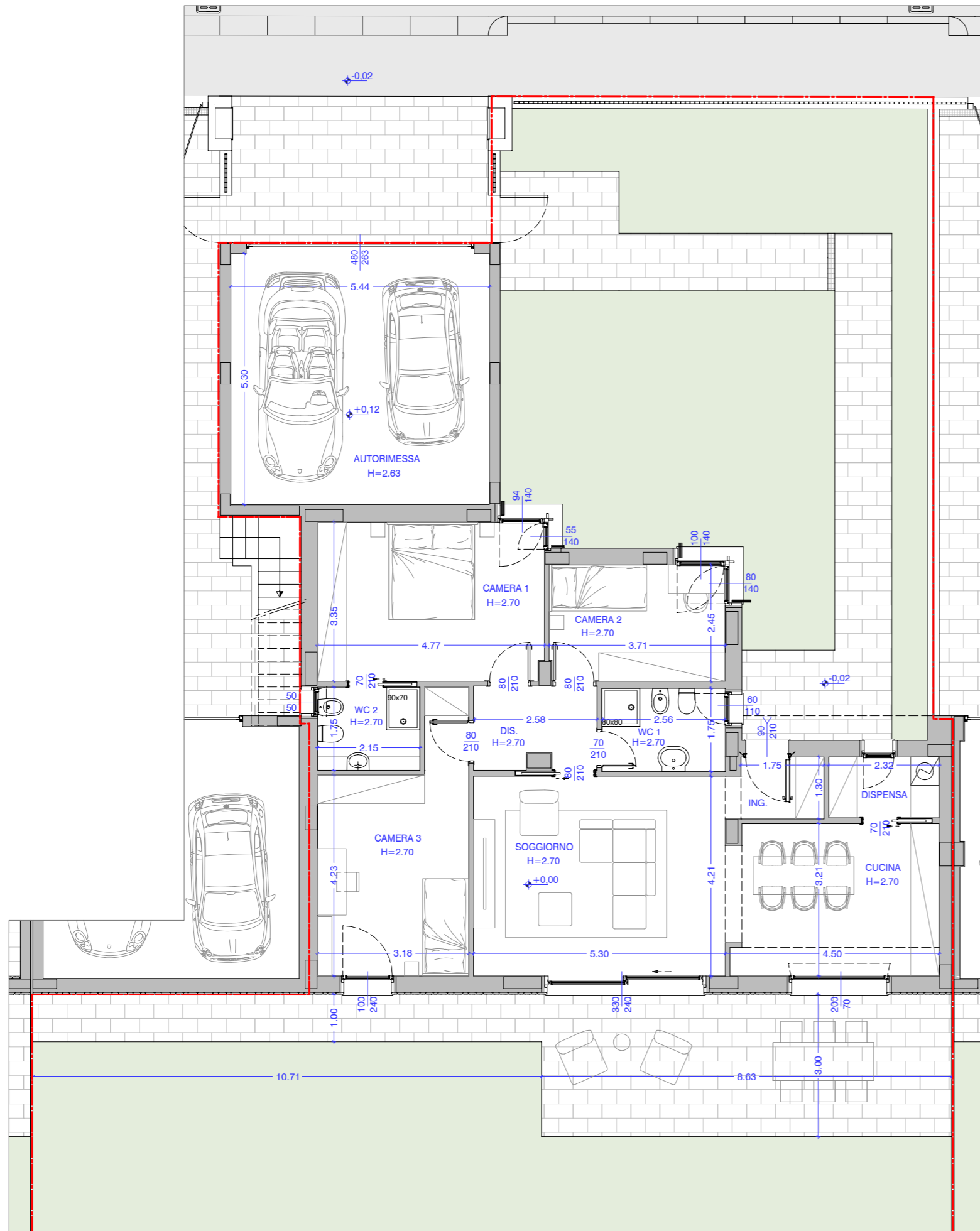
PIANO TERRA_scala 1:100
